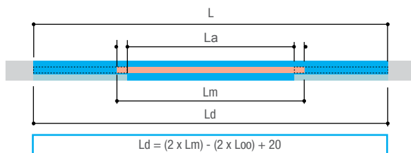
DVOKRILNA KLIZNA VRATA
